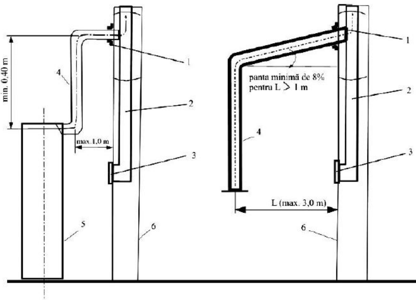
Fig. 13 Racordarea la coș de fum cu burlane
